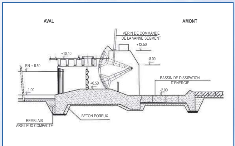
COUPE TYPE
