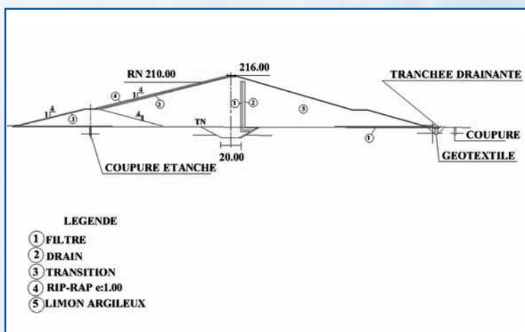
COUPE TYPE
